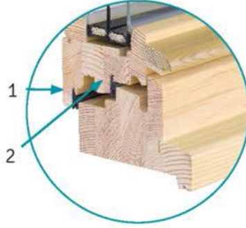
2 joints d'étanchéité
