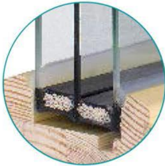
Intercalaire Warm Edge ou Swisspacer V
