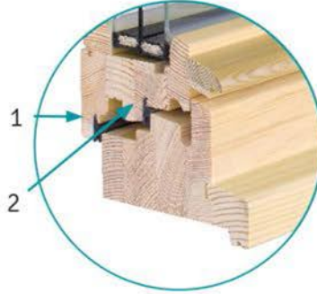
2 joints d'étanchéité
