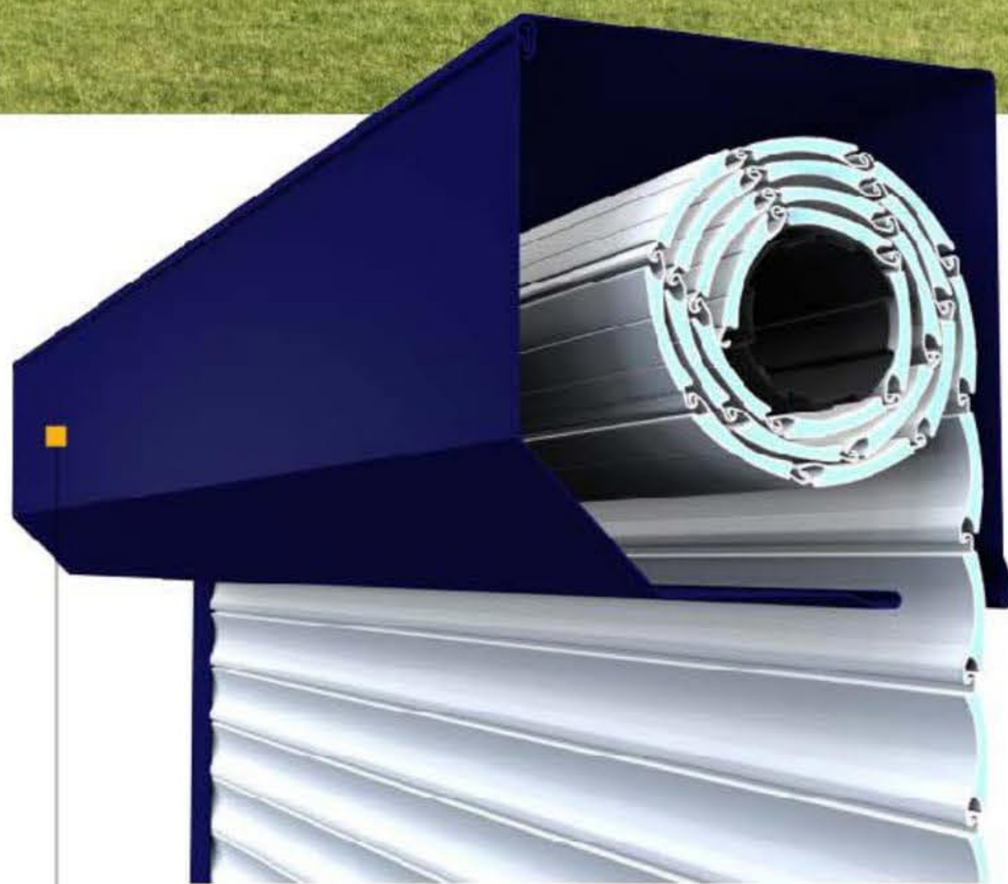
Coffre extérieur CLASSIQUE avec pan coupé
