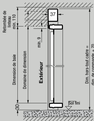
Coupe verticale
