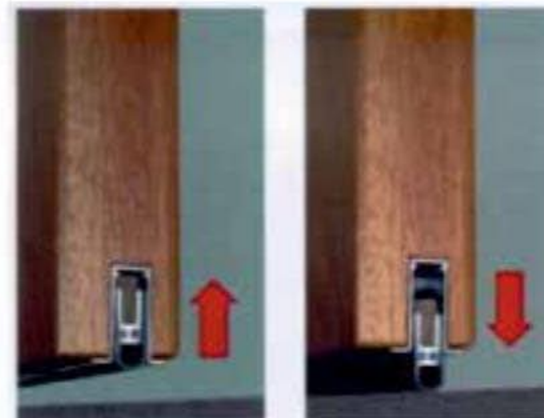
SEUIL MÉCANIQUE SOULEVABLE INTÉGRÉ AU VANTAIL
