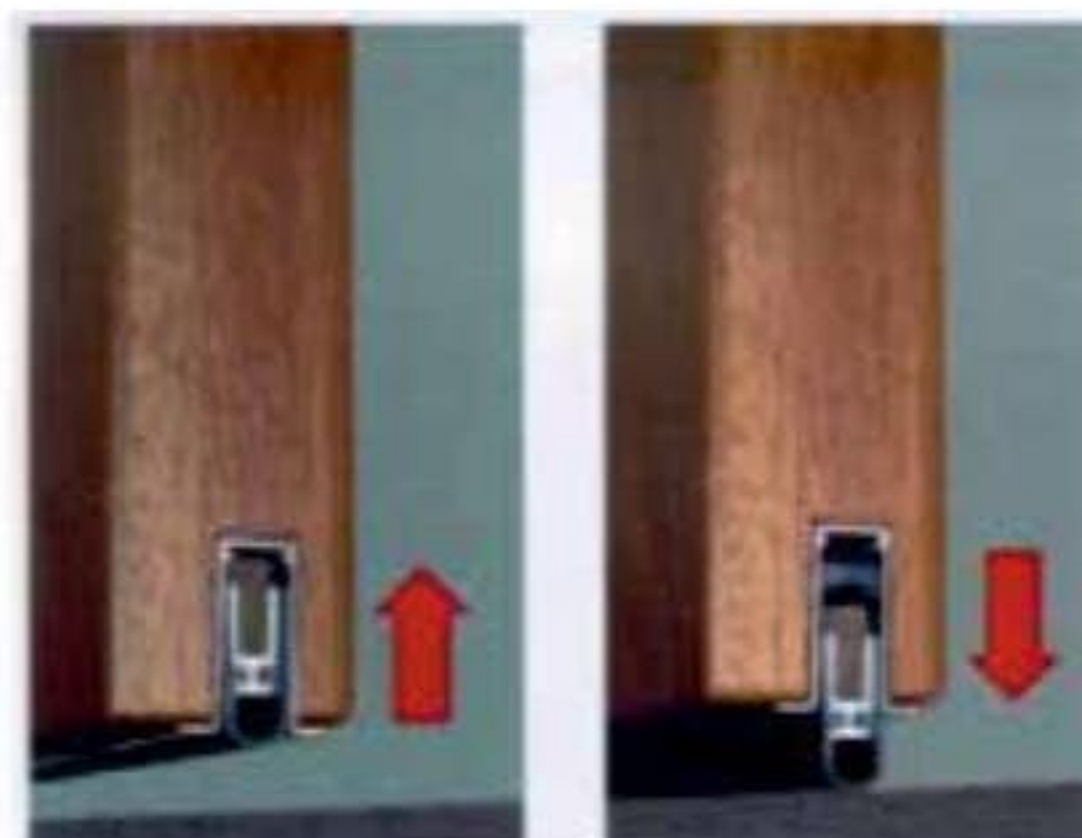
SEUIL MÉCANIQUE SOULEVABLE INTÉGRÉ AU VANTAIL
