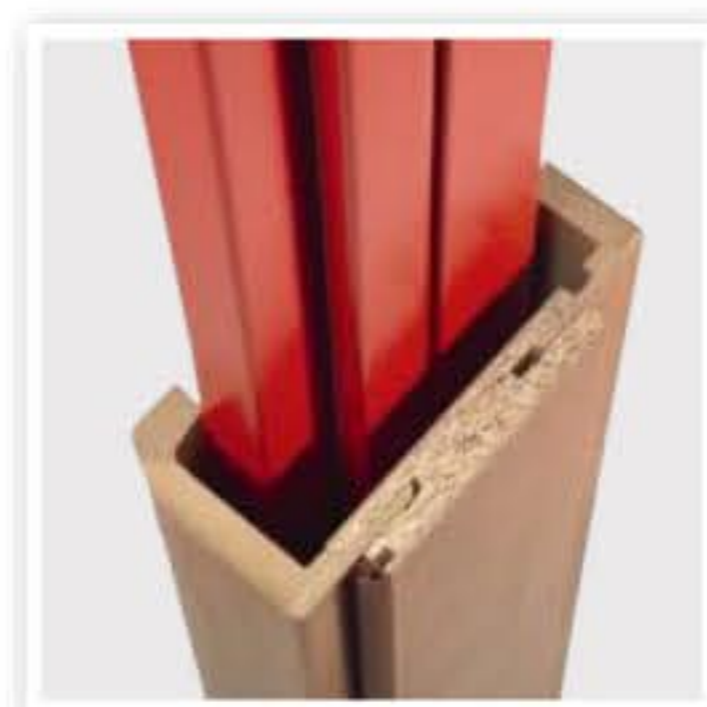
▲ Largeur d'habillage 85 mm, galbé, retour coudé de 20 mm
