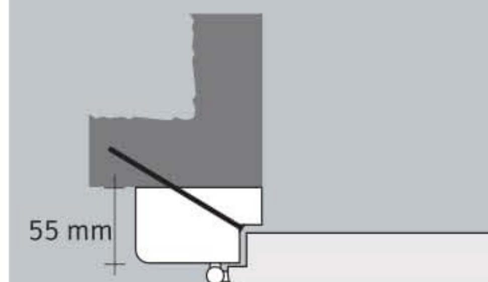
▲ Bloc porte en applique
